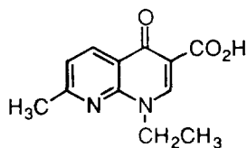
nalidixic acid
